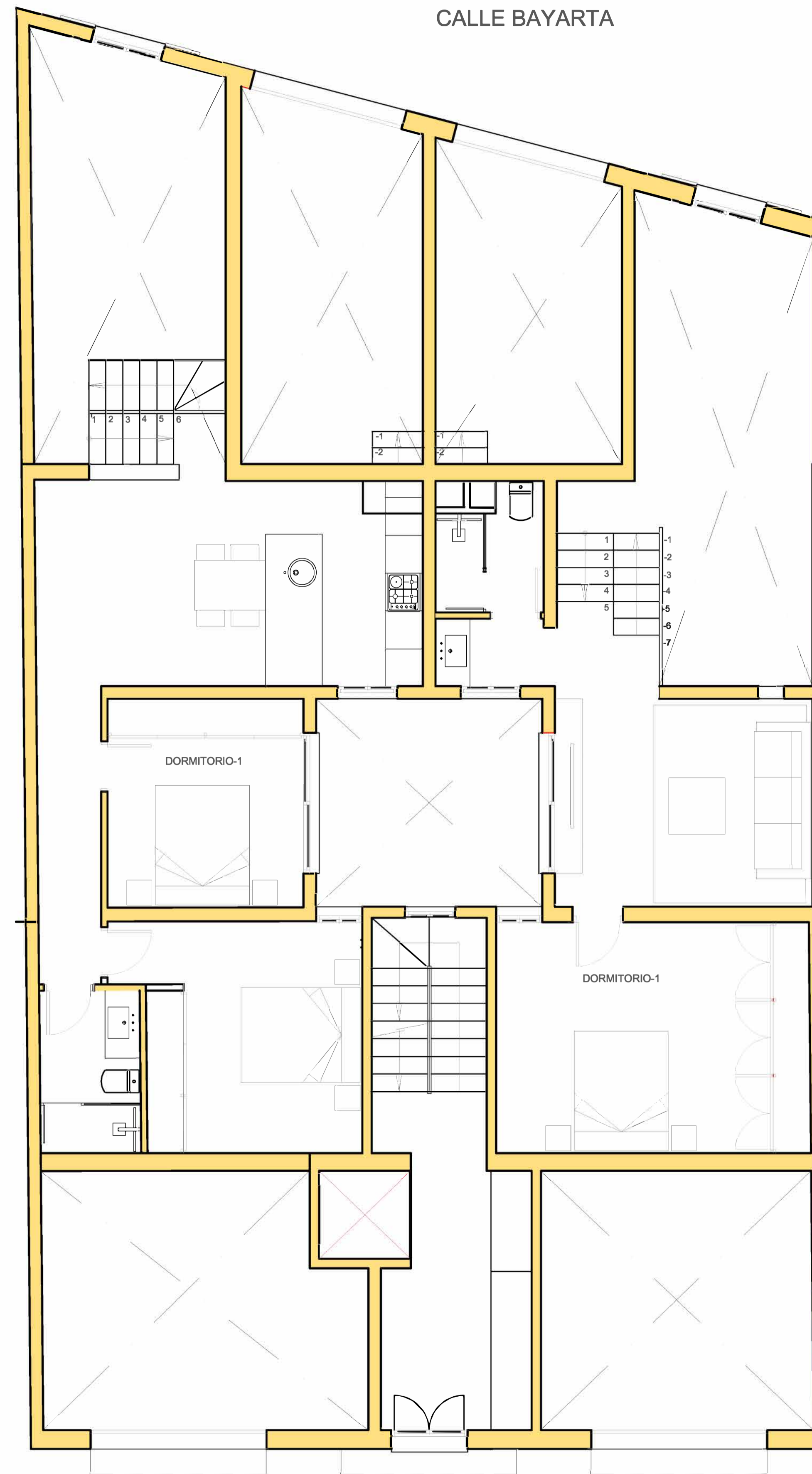
PLANTA ALTILLO PLANTA cota +1,10m
