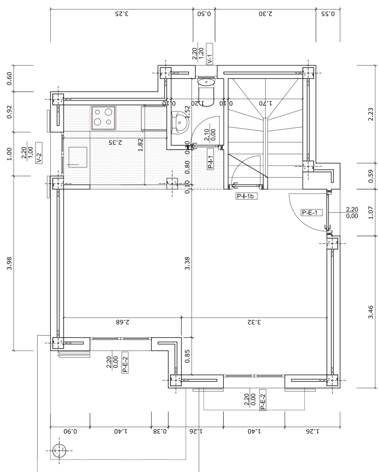
UNTERGESCHOSS
