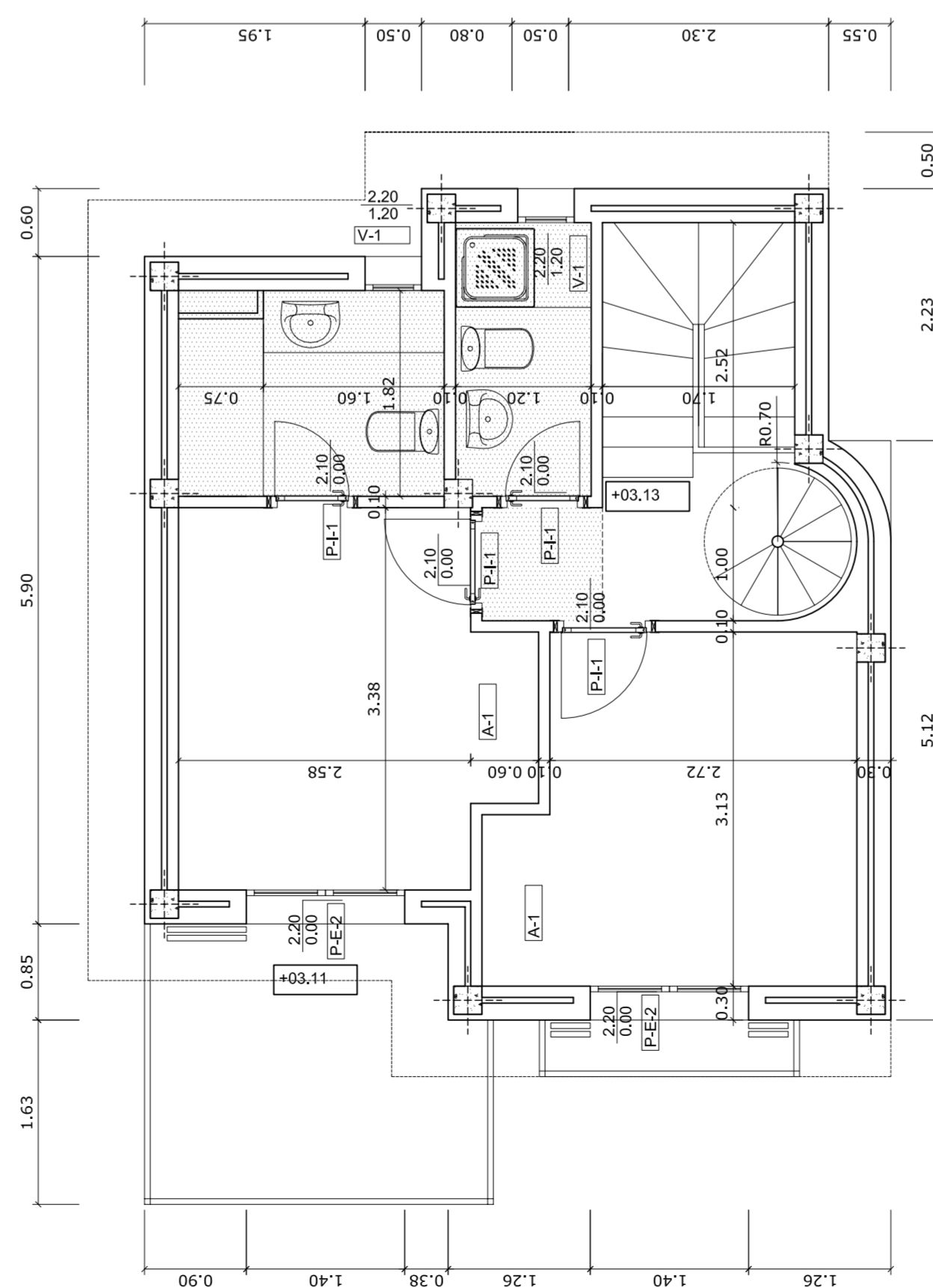
OBERGESCHOSS
