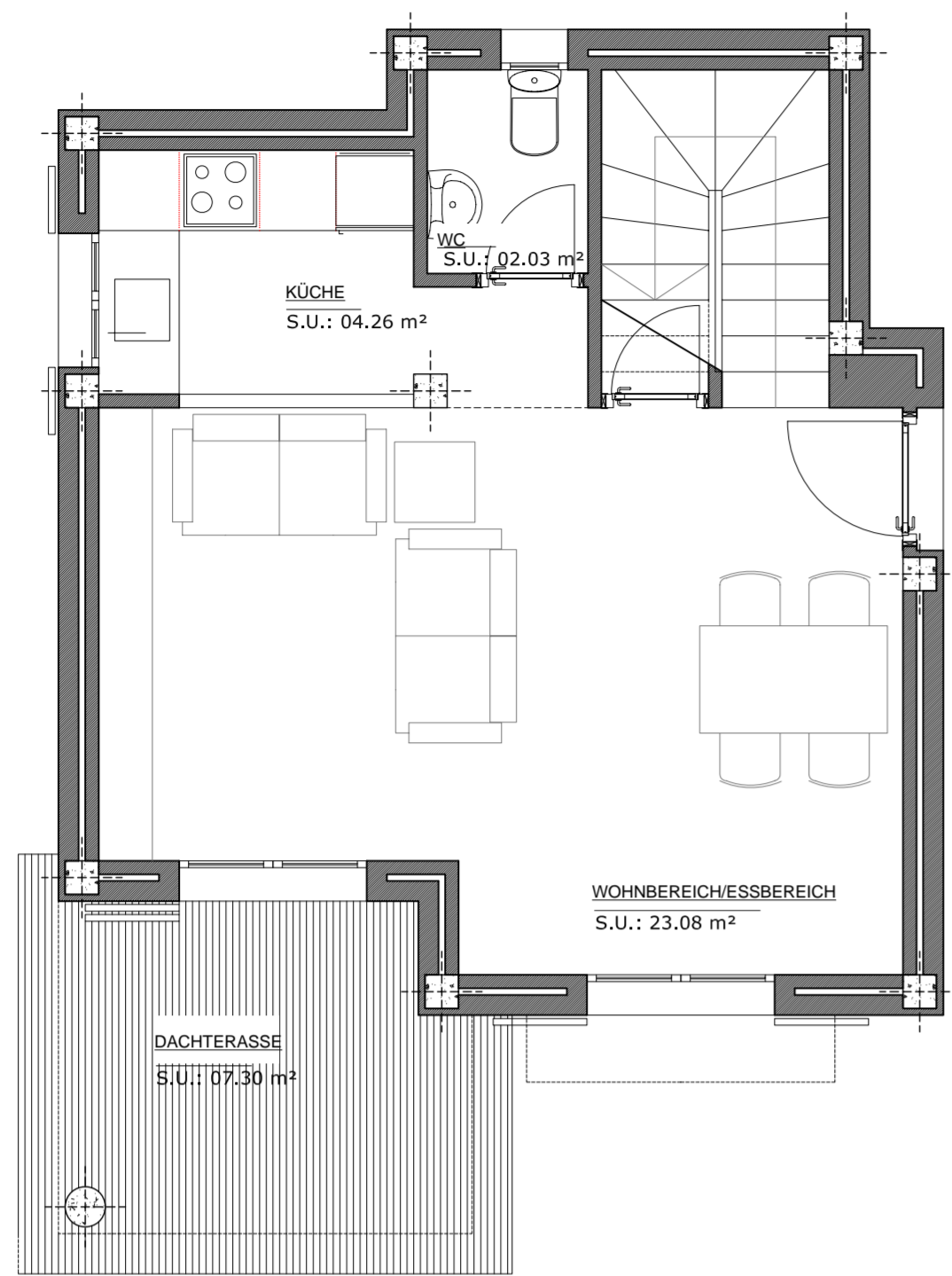
UNTERGESCHOSS
