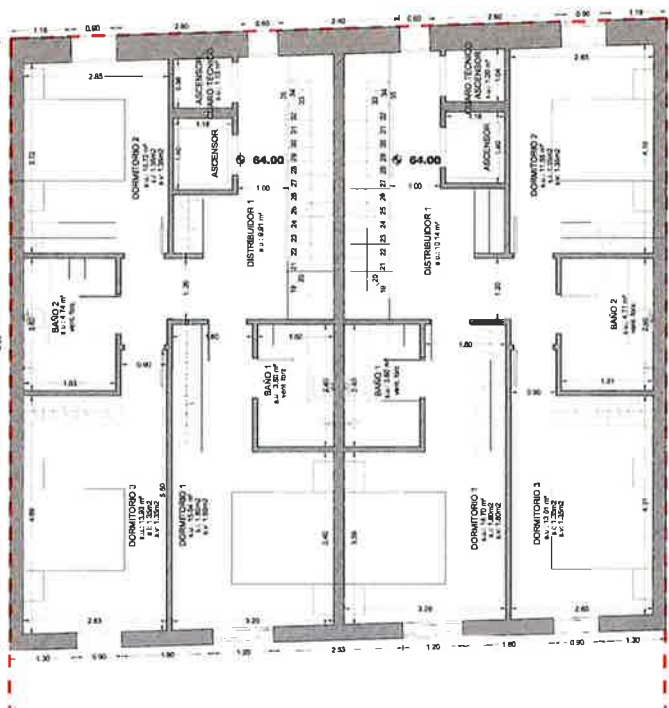
VIVIENDA C Y VIVIENDA D PLANTA PRIMERA
