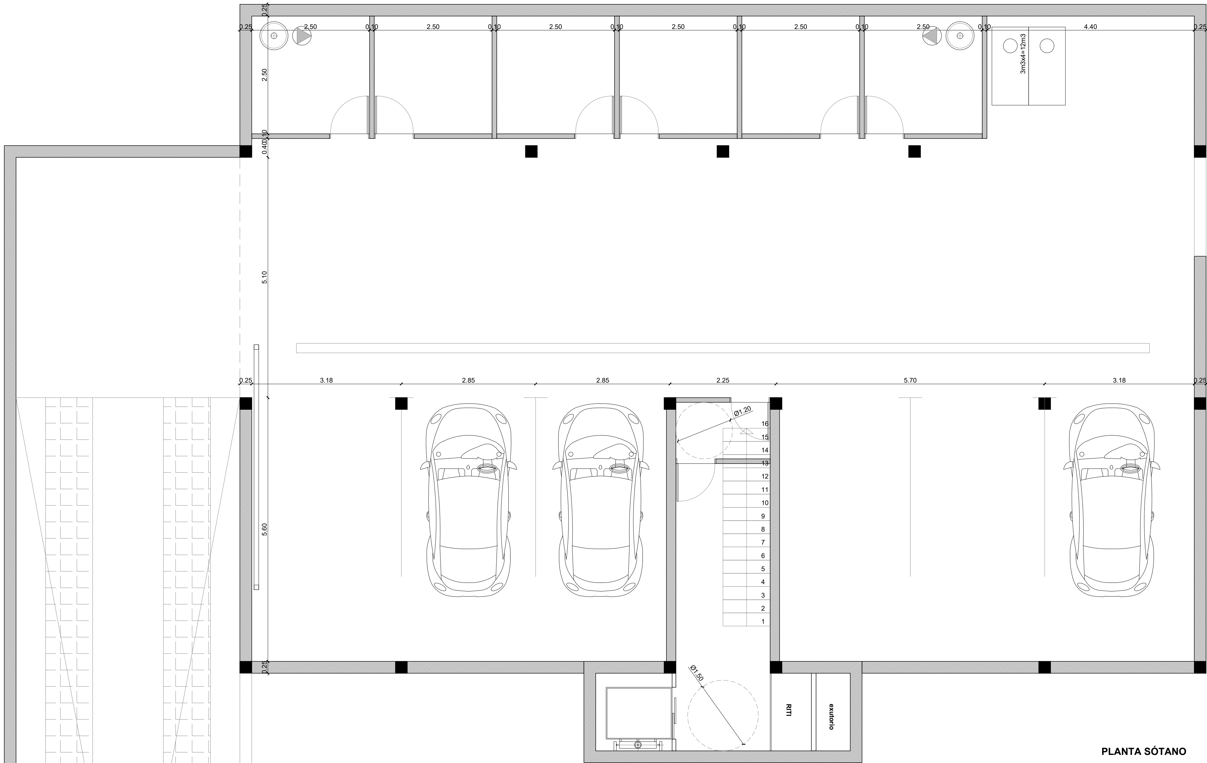
PLANTA SÓTANO
