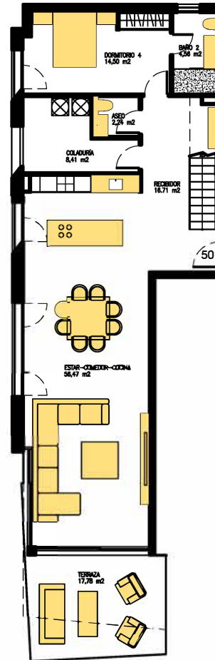
PLANTA BAJA
